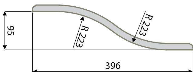
FRONT GIĘTY TYP S L
