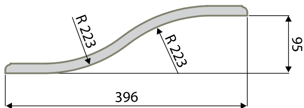
FRONT GIĘTY TYP S P
