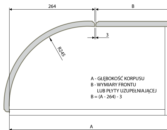
SPOSÓB OBLICZENIA FRONTU LUB FORMATKI UZUPEŁNIAJĄCEJ DO SZAFEK DOLNYCH PRZY WYKORZYSTANIU FRONTU GIĘTEGO Z PROMIENIEM ZEWNĘTRZNYM
