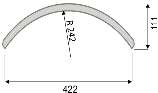
FRONT GIĘTY TYP S L
