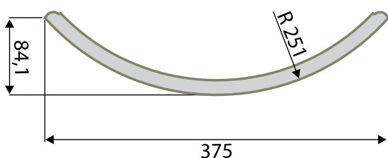
FRONT GIĘTY WEWNĘTRZNI
