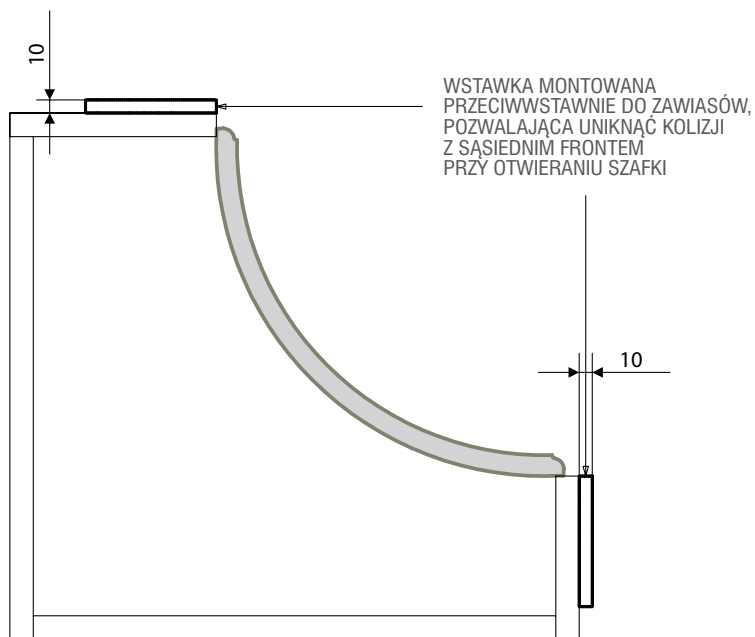
POPRAWNE ZAMONTOWANIE FRONTU GIĘTEGO WEWNĘTRZNEGO, POZWALAJĄCE UNIKNĄĆ KOLIZJI PRZY OTWIERANIU SZAFKI,
