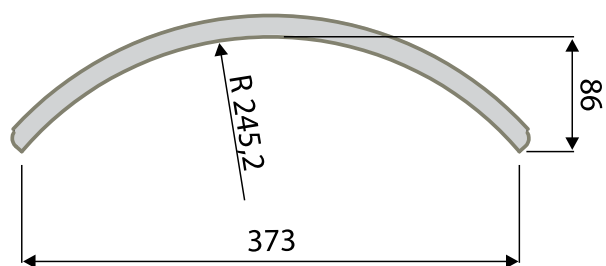
FRONT GIĘTY ZEWNĘTRZNI
